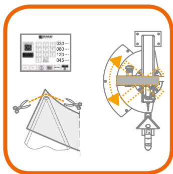
Regolazione dell'angolo di taglio elettronico Adjustment of electronic cutting angle
