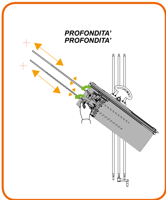
Dispositivi per il posizionamento e la messa in taglia delle maniche, regolabili dall'operatore velocemente Positioning and sizing device for sleeve, quickly adjustable by the operator
